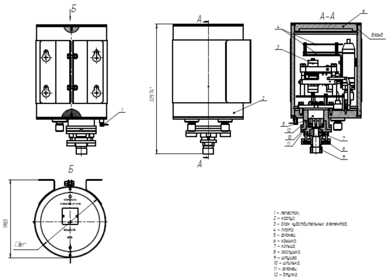
Рисунок 12 - Преобразователь ледяный внешний вид
