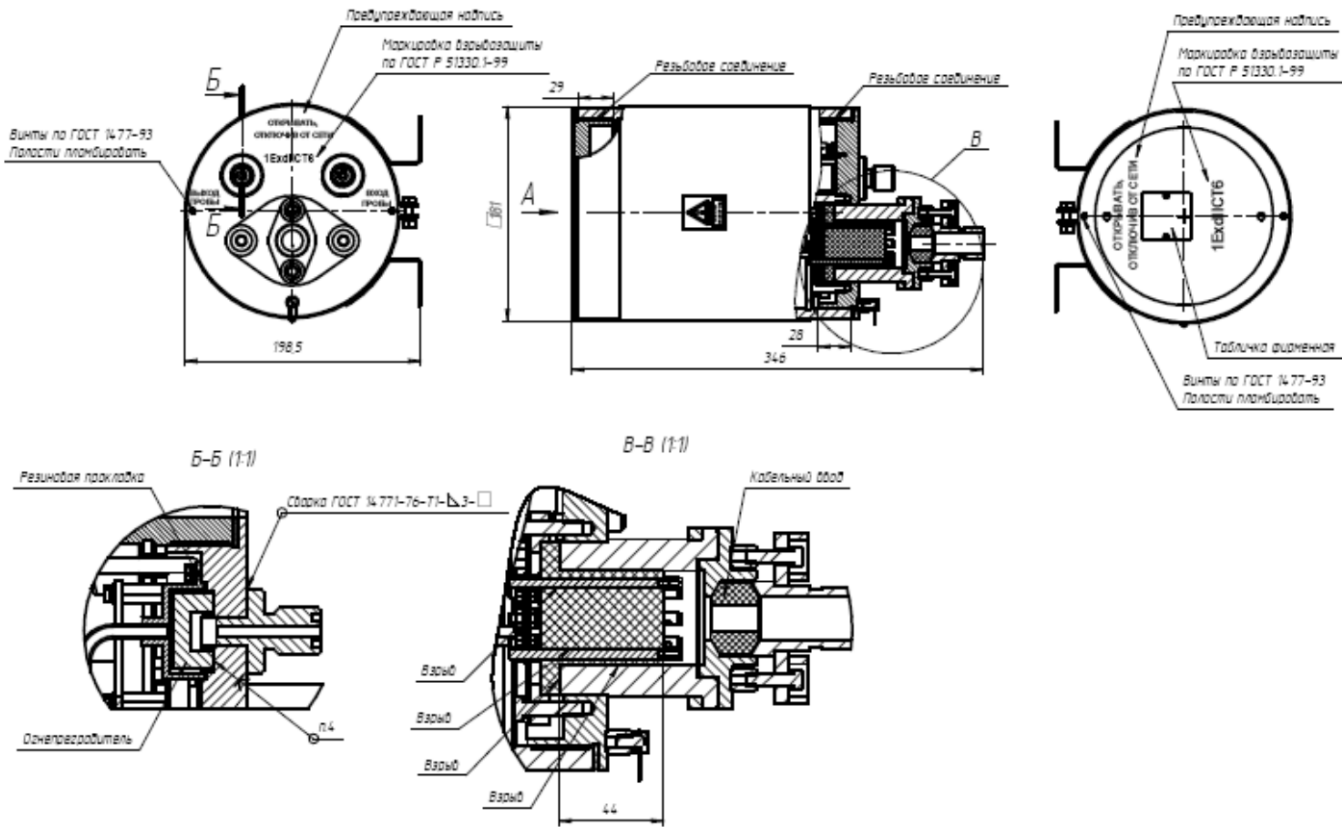
Чертеж средств взрывозащиты Рисунк 2 (для исполнения ПИЛ ПБ/Д407111004-04 -09) Остальное - см. дис 1
