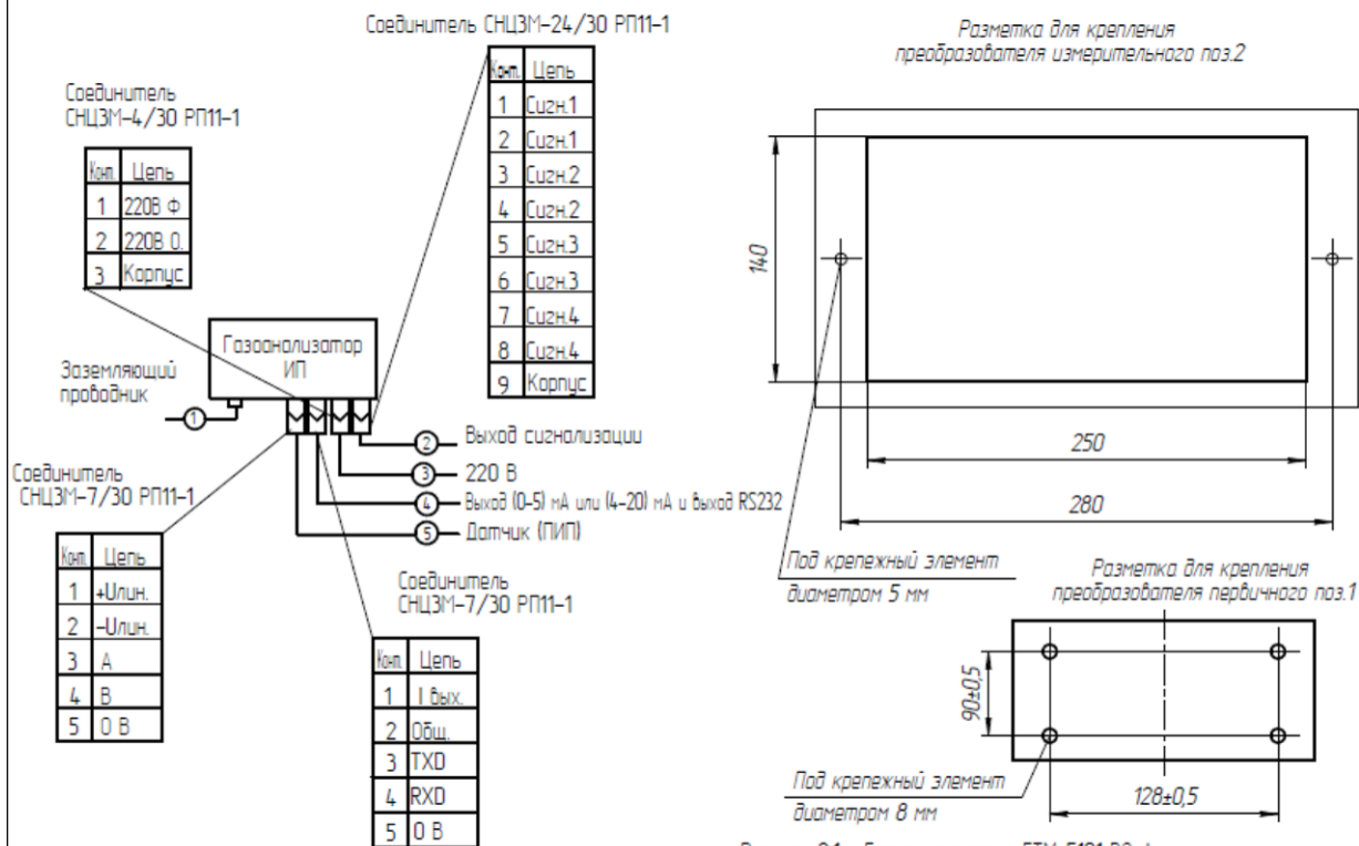
Рисунок 2.1 – Газоанализаторы ГТМ-5101 ВЗ-А. Схема внешних электрических соединений
