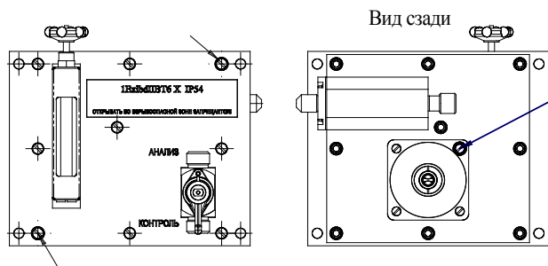
Рисунок Г.2 - ВД сигнализаторов STM-30M-04ПЦВ, -53ПБВ с принудительным отбором пробы
